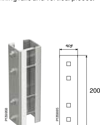
Pendant joint 20J
