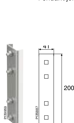
Pendant joint 2J
